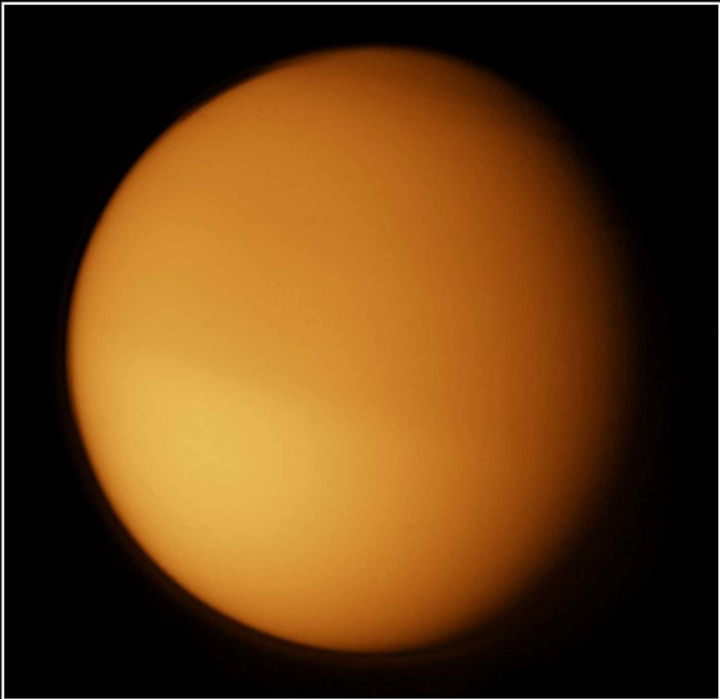
Titan
